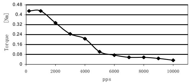
FL57ST51-0856A
