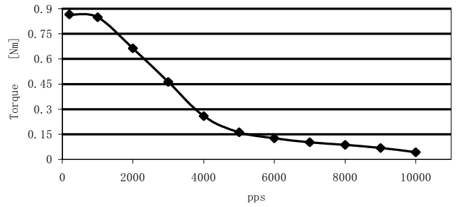
FL57STH76-1506A
