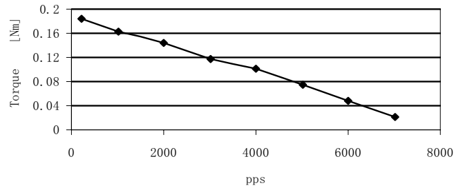
FL57ST51-0856A
