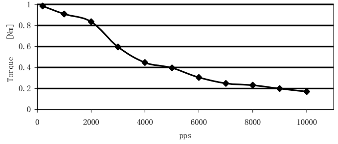
FL57STH76-2006MA
