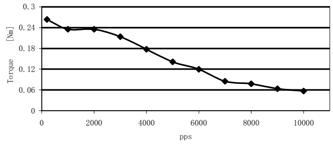
FL42STH47-0806A
