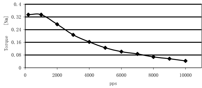
FL42STH47-1684MA
